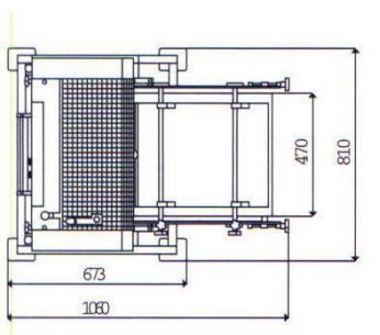
Rollomat s dovalovací deskou Za příplatek, pro větší výrobu vek apod.
